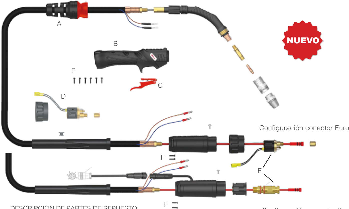
Configuración conector tipo Tweco
